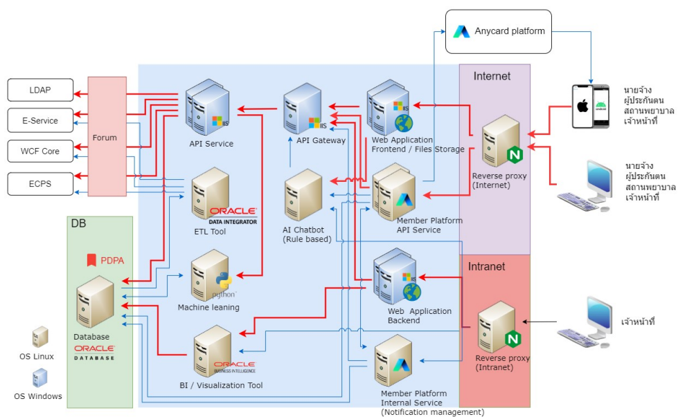
ภาพที่ 2 SYSTEM ARCHITECTURE
